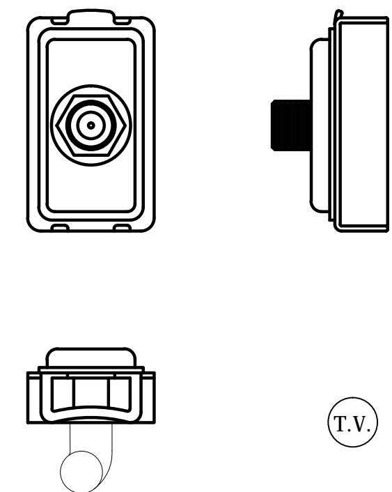
CONECTOR TV BTICINO 5152E ESCALA 1:1
