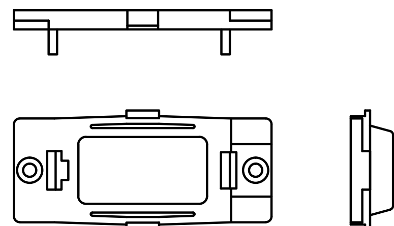
SOPORTE P/PLACA TABIQUE 12579 ESCALA 1:1
