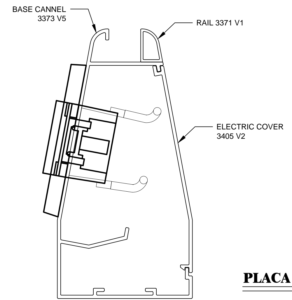
ASSEMBLY 2 - TOMA DEC. SIN TORN. ESCALA 1:1
